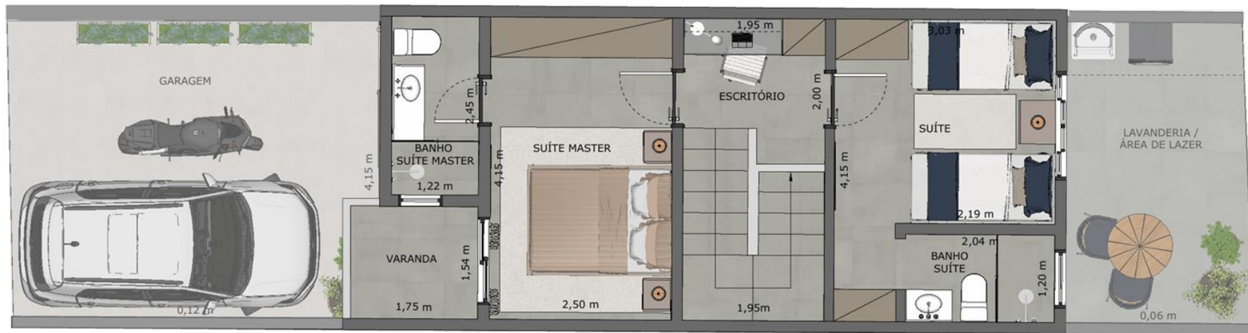
PAVIMENTO SUPERIOR
